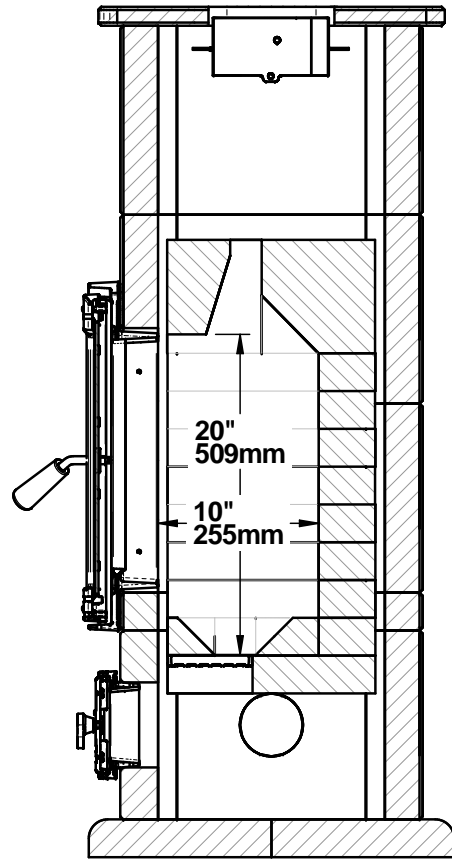
SECTION A-A
